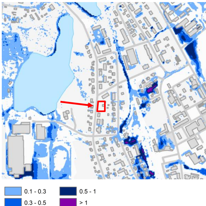
Figur 16. Översvämningskartering som visar det beräknade maximala vattendjupet (m) i samband med 100-årsregn. Källa: DHI (2018).
